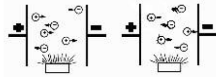
Fig. 3: principio de funcionamiento de detectores iónicos de humos
